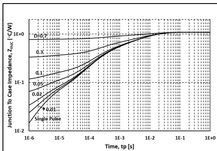
图. 23 热阻曲线
